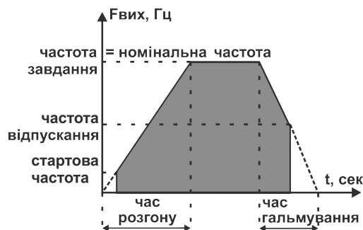
Рисунок 9. Динамічні параметри приводу.
