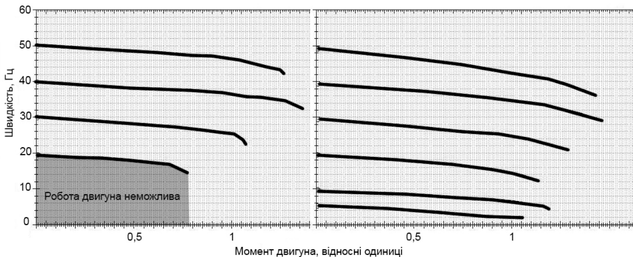
Рисунок 22 а) Механічні характеристики двигуна при підключенні з конденсатором. Рисунок 22 б) Механічні характеристики двигуна при підключенні без конденсатора.
