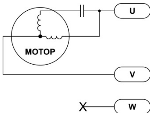
Рисунок 21 а) Підключення однофазного двигуна з конденсатором до ПЧ.
