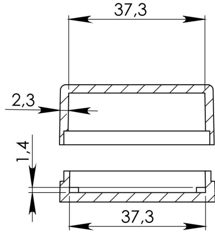
PRZEKRÓJ A-A
